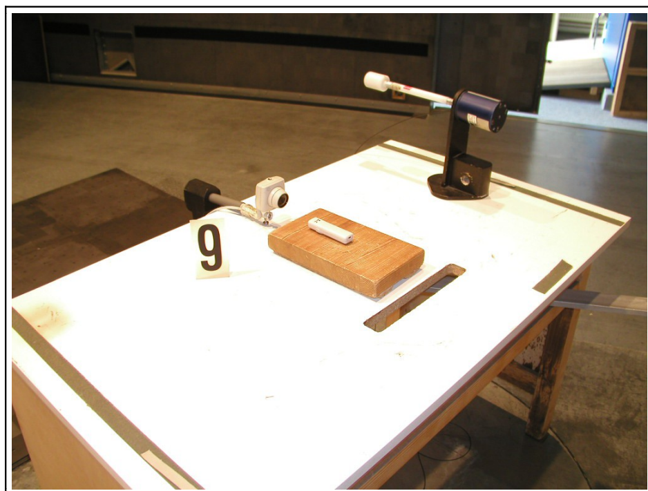
Bild 2 : Prüfanordnung "Funkstörfeldstärkemessung", "Störfestigkeit gegen elektromagnetische Felder"
